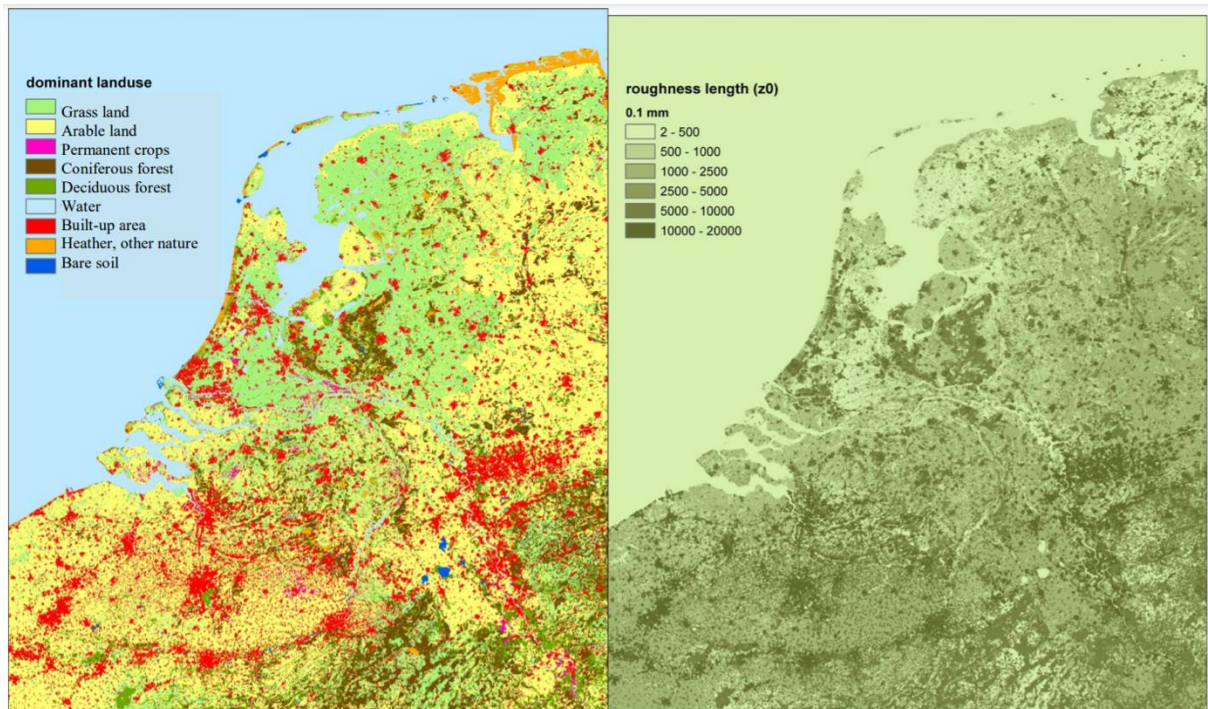
Figuur 45: Dominant landgebruik (volgens DEPAC) en ruwheidslengte op 250 bij 250 m 2 , afgeleid van LGN7 voor Nederland en CLC2006 voor België en Duitsland (volgens handleiding OPS).
